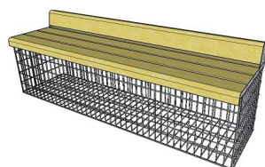
Banc 2.00m Gabion 2.00m Mélèze: E200BI
